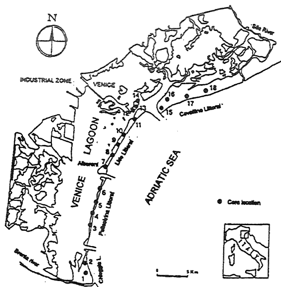
Fig. 1 - Ubicazione dei 18 sondaggi "lito" (da Gatto, 1980a). Borehole location (after Gatto, 1980a).
