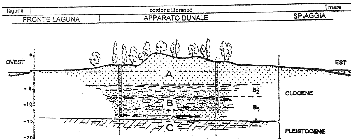
Fig. 6 - Sezione stratigrafia trasversale del litorale di Lido in località Alberoni. Legenda: A) Complesso sabbioso; B) complesso misto; C) complesso pleistocenico limo-argilloso.
