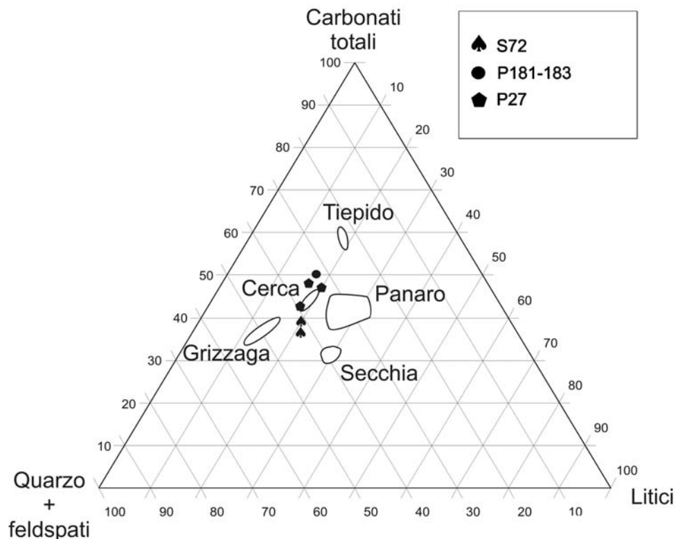
Fig. 10 - Composizione dei campioni prelevati nelle perforazioni TAV con età minore di 10-12 ka. Nel diagramma sono indicati i campi composizionali delle sabbie attuali e recenti (Neolitico) dei corsi d'acqua modenesi.
