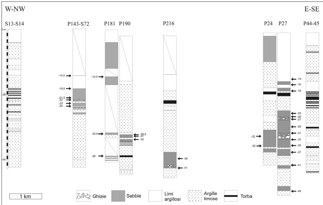
Fig. 9 - Stratigrafie delle perforazioni TAV esaminate (non in scala). Le frecce indicano i campioni di sabbie analizzati. Stratigraphic columns of the studied wells along the TAV track (not to scale). Arrows point to the analyzed sand samples.
