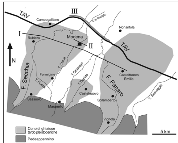
Fig. 1 - Idrografia principale dell'alta e media pianura modenese e traccia del percorso della linea TAV. E' illustrata la distribuzione dei corpi ghiaiosi che costituiscono le conoidi pedemontane tardo-pleistoceniche dei fiumi Secchia e Panaro e del T. Tiepido (modificata da PELLEGRINI & ZAVATTI, 1979). I = sezione geologica di Fig. 4; II = sezione geologica di Fig. 5; III = sezione geologica di Fig. 6.
