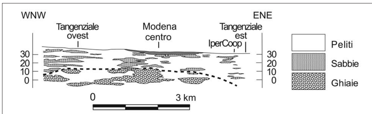
Fig. 5 - Sezione geologica attraverso l'area urbana di Modena (a nord della Via Emilia) nella quale è evidenziata (linea tratteggiata) il limite tra la porzione superiore costituita da peliti e corpi sabbiosi discontinui (Subsistema di Ravenna) e la porzione sottostante ricca in corpi ghiaioso-sabbiosi (unità di Vignola). In corrispondenza del centro cittadino è evidenziata l'unità di Modena (puntinato) con depositi di epoca post-romana (modificata da FAZZINI & GASPERI, 1996).
