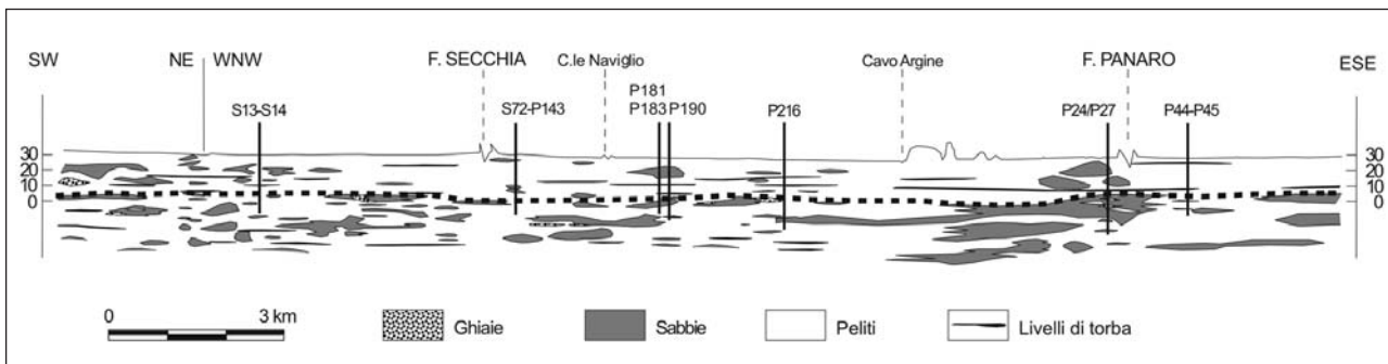
Fig. 7 - Sezione stratigrafica lungo il tracciato della linea TAV (modificata da VALLONI et al. , 2003). La linea tratteggiata indica il limite fra la porzione superiore (Subsistema di Ravenna) e la porzione sottostante (unità di Vignola). Sono indicate le perforazioni dalle quali sono stati prelevati i campioni di sabbie analizzati.
