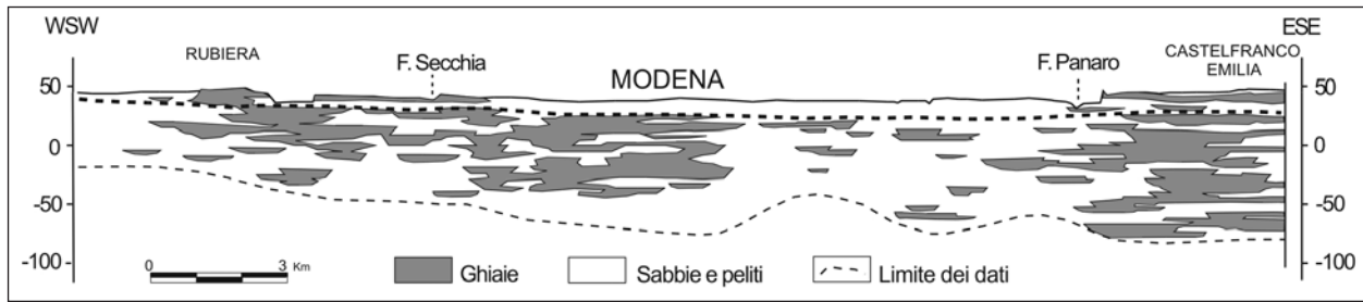
Fig. 4 - Sezione geologica trasversale alla pianura modenese passante a sud del centro urbano che evidenzia la distribuzione in profondità dei corpi ghiaiosi (da GASPERI et al. , 1989). La linea tratteggiata in grassetto divide la parte superiore, con scarsi corpi ghiaiosi (Subsistema di Ravenna) da quella inferiore, caratterizzata da un notevole sviluppo di depositi grossolani. La linea tratteggiata inferiore rappresenta il limite dei dati.
