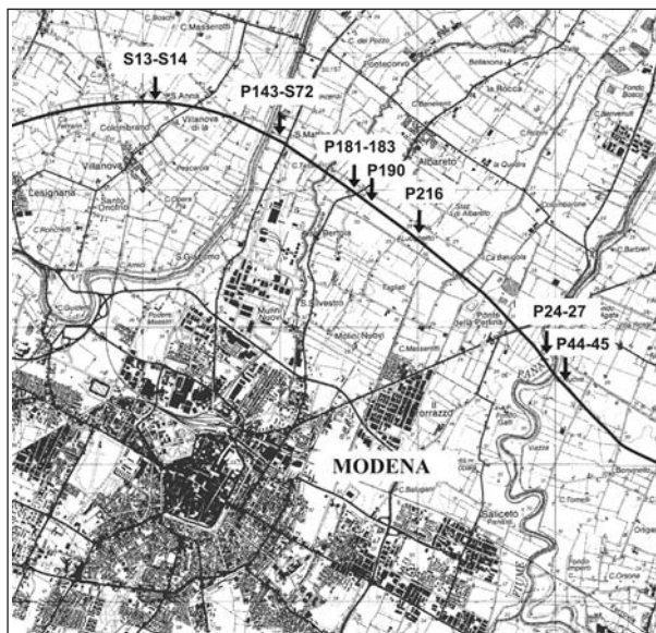
Fig. 8 - Ubicazione delle perforazioni studiate lungo il tracciato ferroviario ad Alta Velocità.
