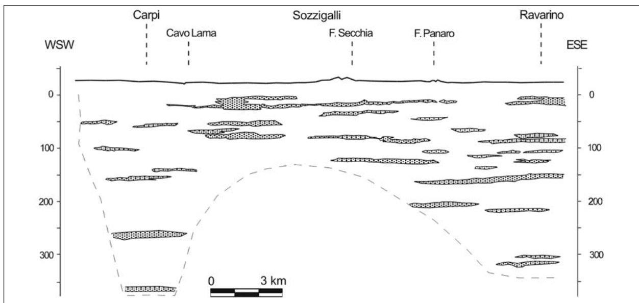
Fig. 6 - Sezione stratigrafica trasversale della pianura modenese all'altezza di Carpi e Ravarino. La sezione è ubicata circa 7 km a nord del tracciato della linea TAV. Sono messi in evidenza i rari e discontinui corpi sabbiosi intercalati a peliti (da: GRUPPO DI STUDIO SULLE FALDE ACQUIFERE DELLA PIANURA PADANA, 1979).
