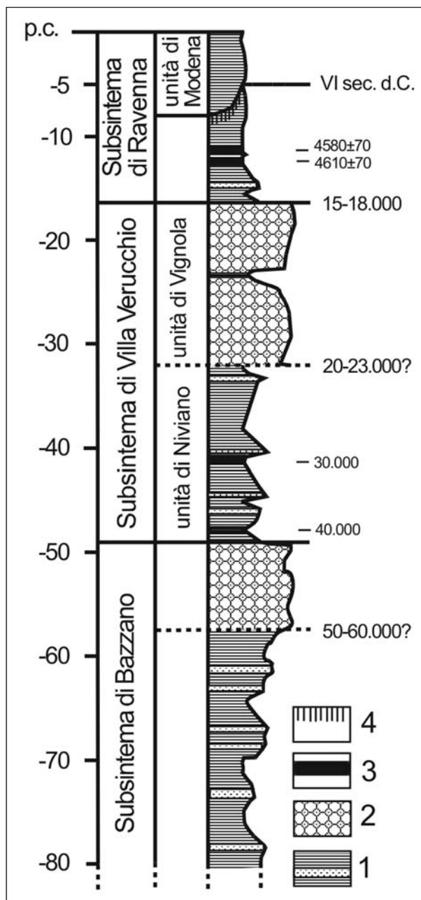
Fig. 3 - Colonna stratigrafica schematica del sottosuolo nel centro urbano di Modena secondo i dati di CREMASCHI & GASPERI (1989) e GASPERI & PIZZILO (in stampa). Legenda: 1) peliti prevalenti con orizzonti sabbiosi; 2) corpi ghiaioso-sabbiosi; 3) livelli con resti organici; 4) orizzonte pedogenizzato.
