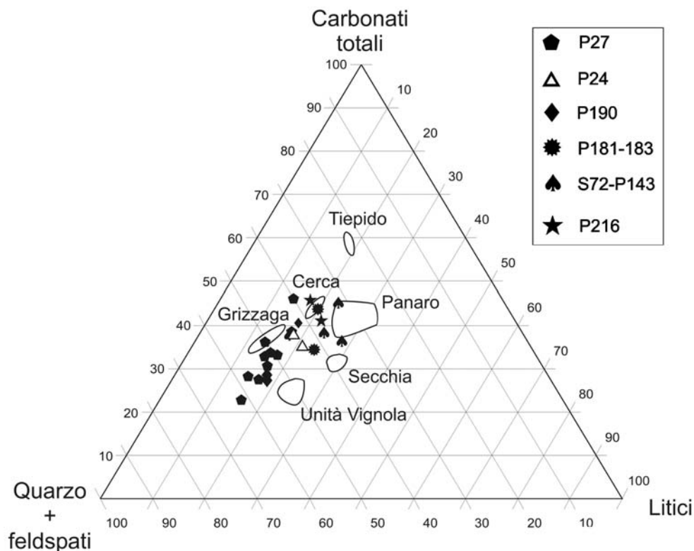
Fig. 11 - Composizione dei campioni prelevati nelle perforazioni TAV con età maggiore di 10-12 ka. Nel diagramma sono indicati i campi composizionali delle sabbie attuali e recenti (Neolitico) dei corsi d'acqua modenesi e dell'unità di Vignola (Pleistocene Sup., presso Formigine).
